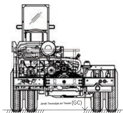
Tampak Belakang
