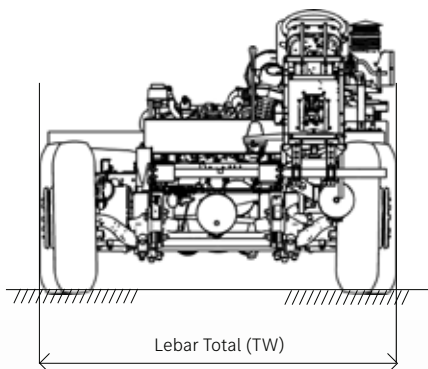
Tampak Depan
