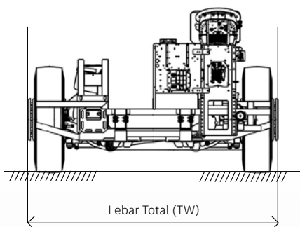
Tampak Depan
